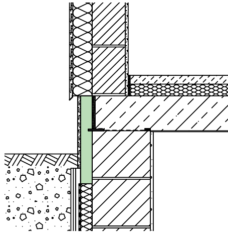
WDVS Wandkonstruktion
