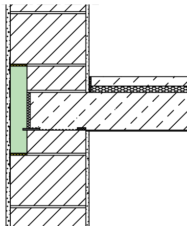
Monolithische Wandkonstruktion
