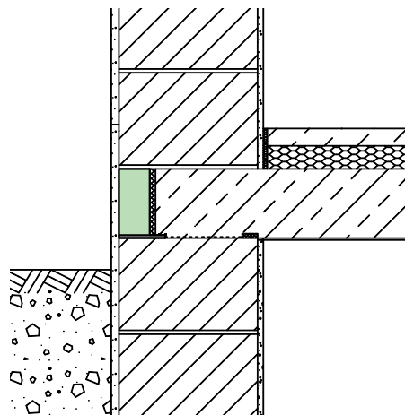
Monolithische Wandkonstruktion
