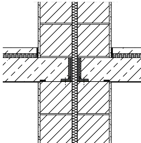
Haustrennwände
