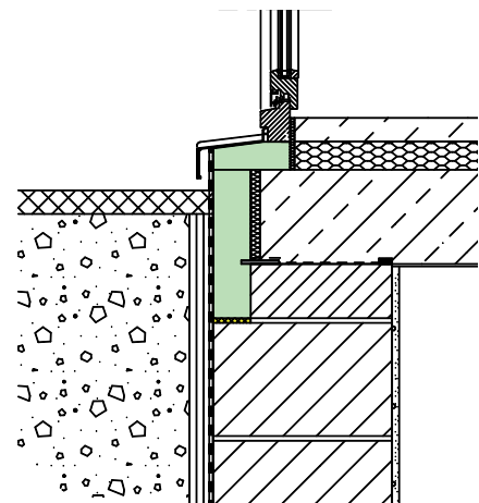
Monolithische Wandkonstruktion
