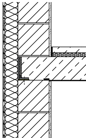
WDVS Wandkonstruktion
