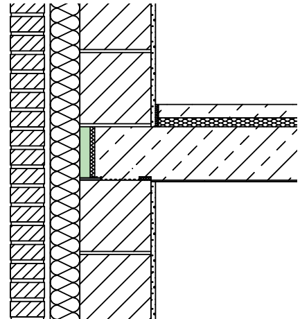
Mehrschalige Wandkonstruktion
