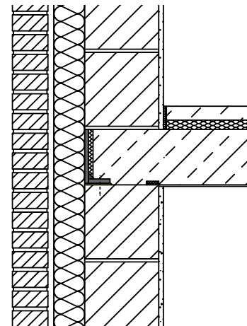
Mehrschalige Wandkonstruktion
